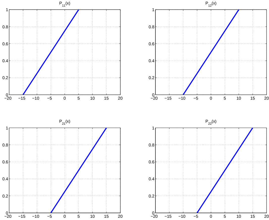
Figura 3.4: Funções cumulativas de probabilidade associadas aos genes de uma população quântica.
