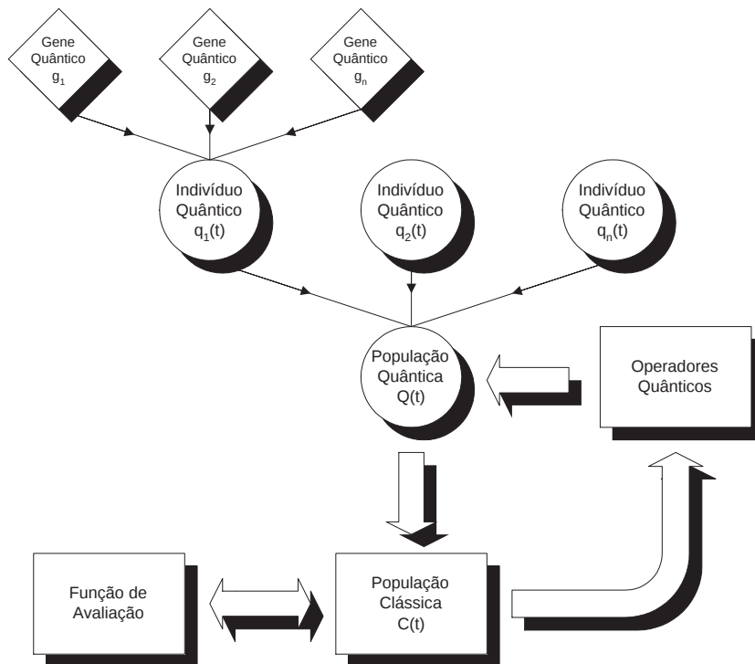
Figura 3.5: Diagrama completo do Sistema Evolutivo com Inspiração Quântica
