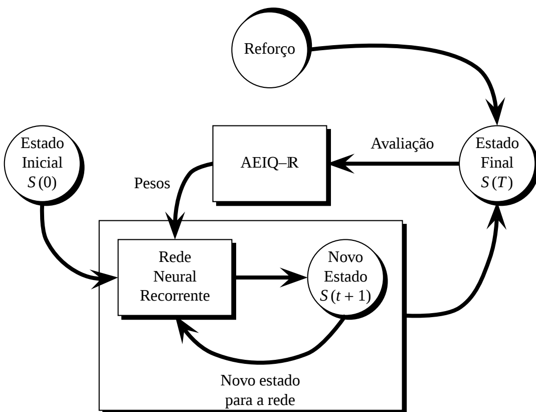
Figura 3.10: Modelo de Aprendizado por Reforço usando o AEIQ–R.
