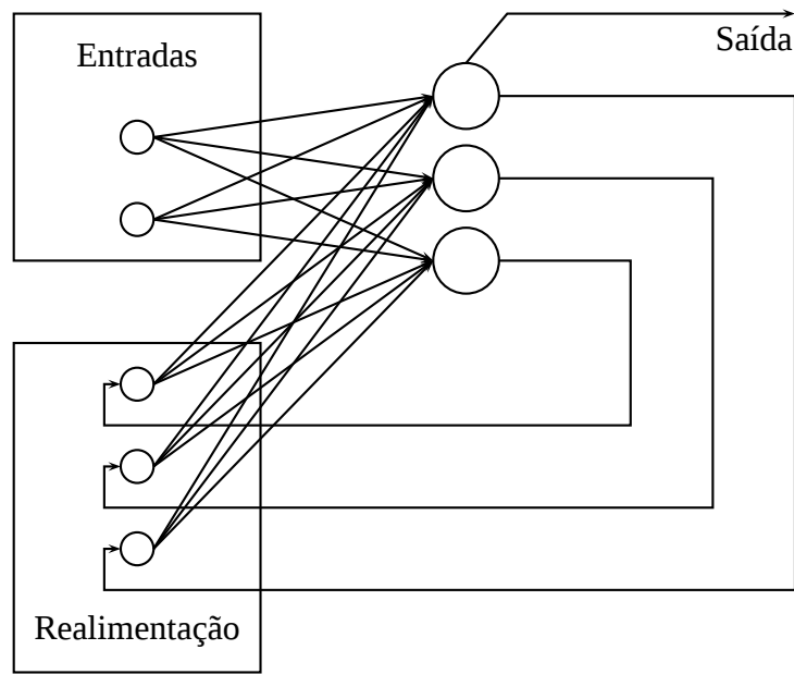
Figura 3.8: Diagrama mostrando uma rede neural recorrente. Este diagrama não mostra as ligações dos biases .
